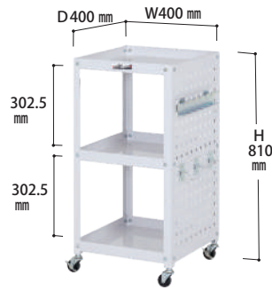
WCLP-3-P 質量：12.0kg ¥44,350(税抜)
