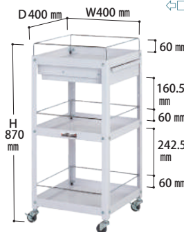
WCLFC-3-P ¥55,100(税抜) 質量：13.1kg
