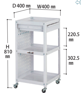
WCLPC-3-P ¥59,350(税抜) 質量：15.0kg
