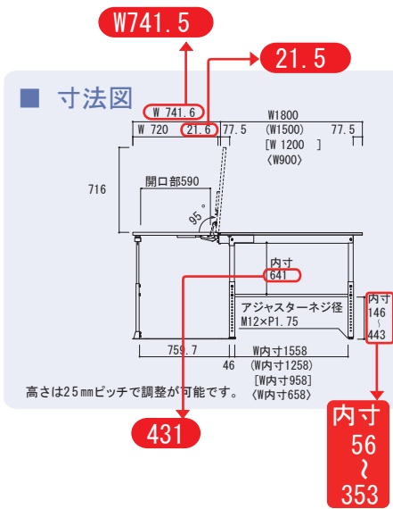
P 64（寸法図内寸法）150 シリーズ跳ね上げタイプ
