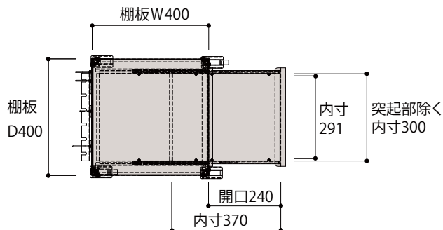
平面図
