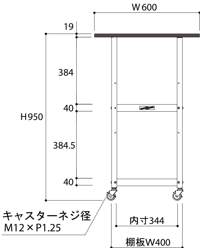
正面図
