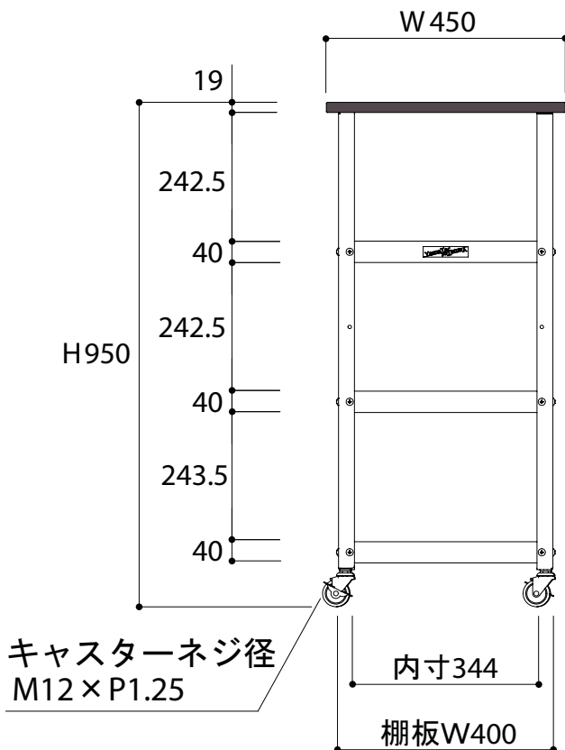
正面図
