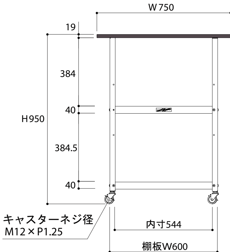
正面図
