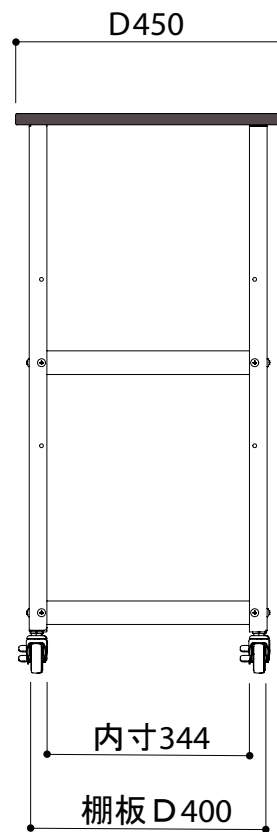
側面図
