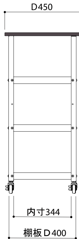
側面図
