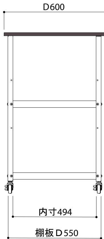
側面図
