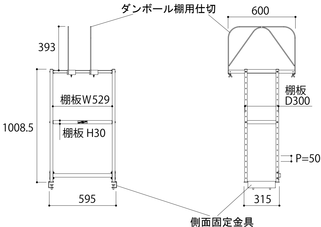
正面図
