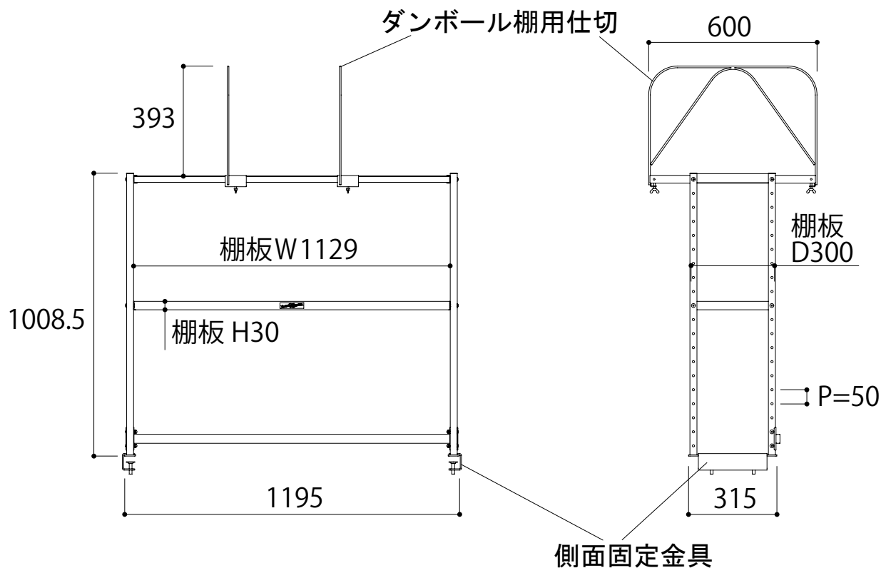
正面図
