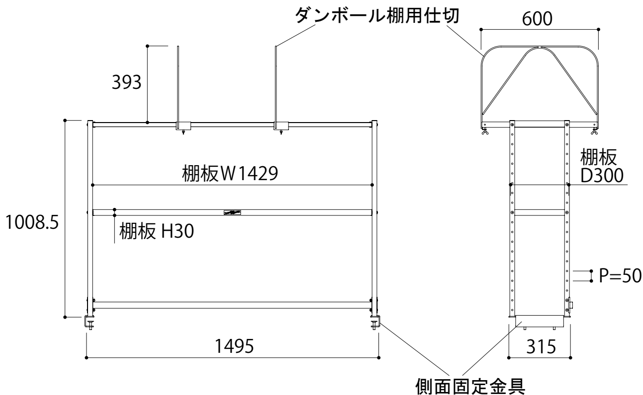
正面図
