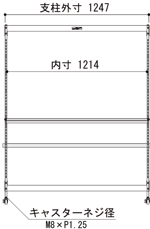
正面図
