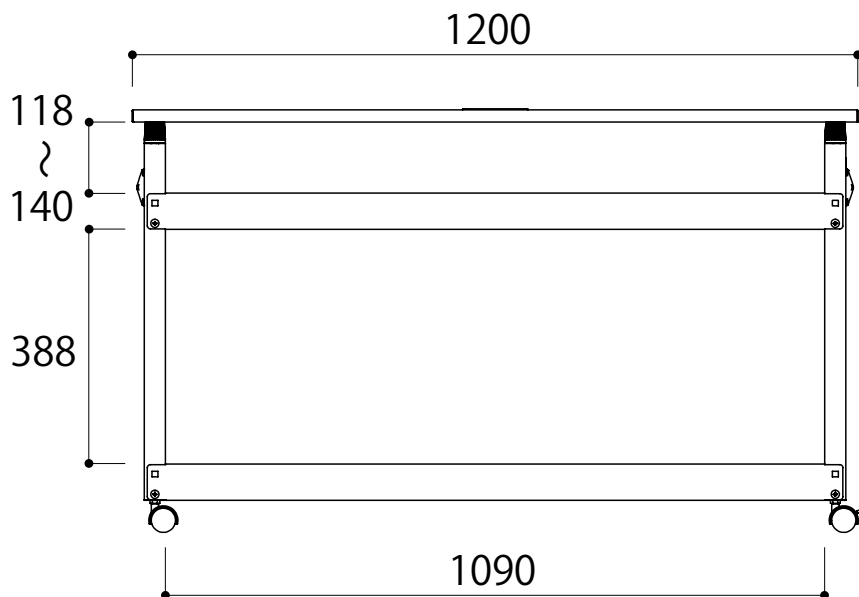
正面図
