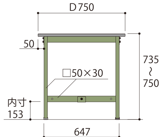
側面図
