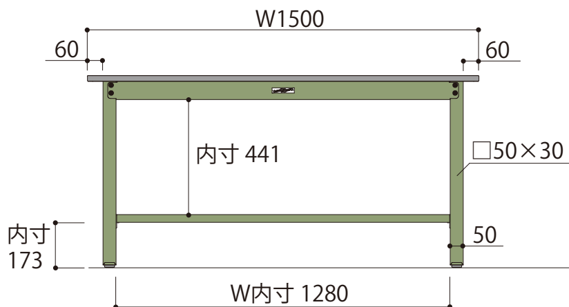
正面図
