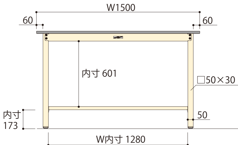
正面図
