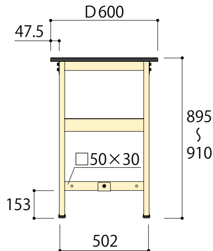
側面図
