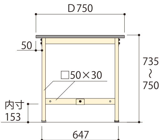
側面図
