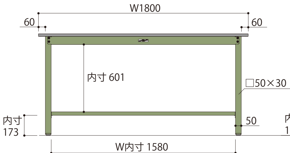
正面図
