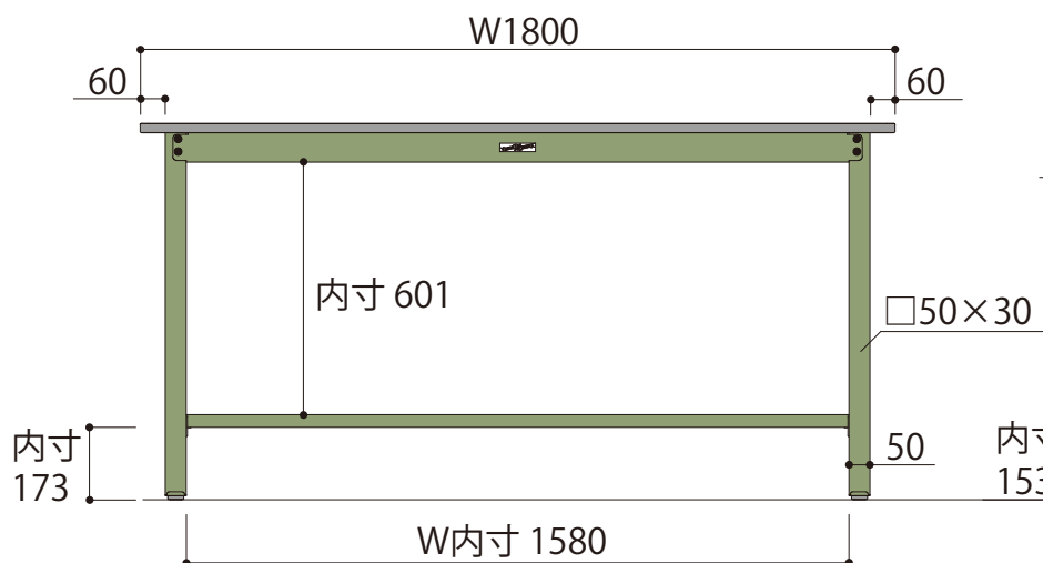
正面図
