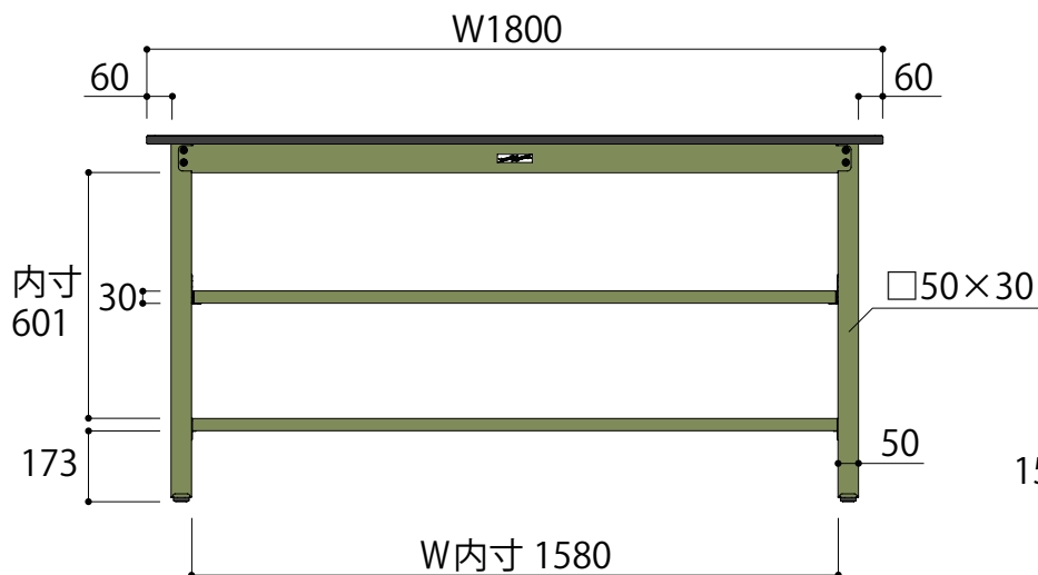
正面図
