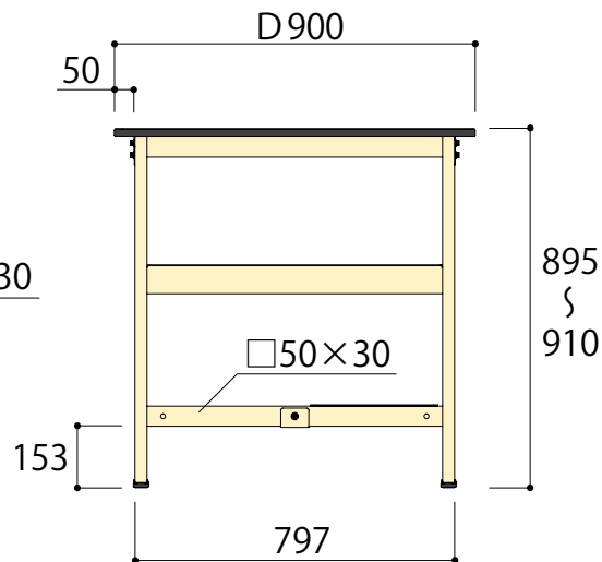
側面図
