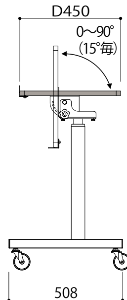
側面図
