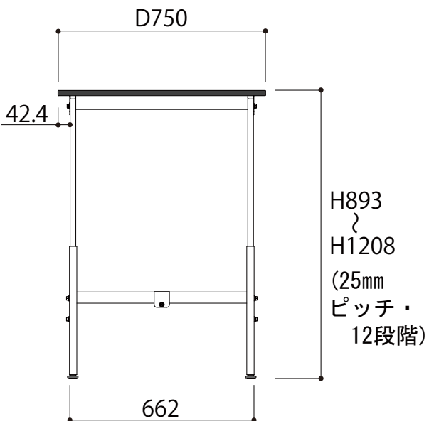
側面図
