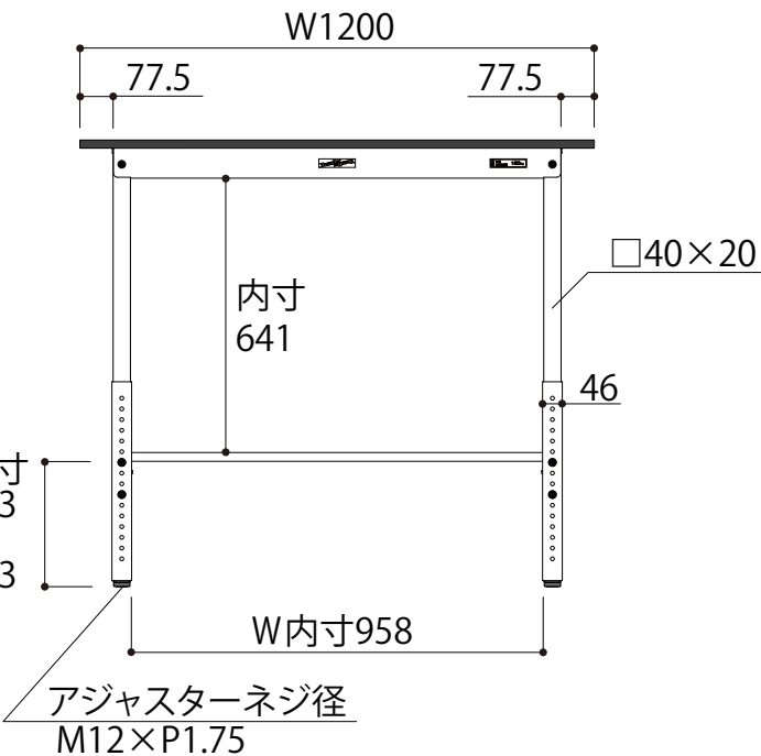
正面図
