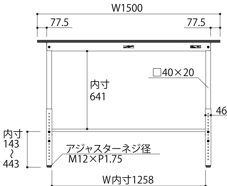
正面図
