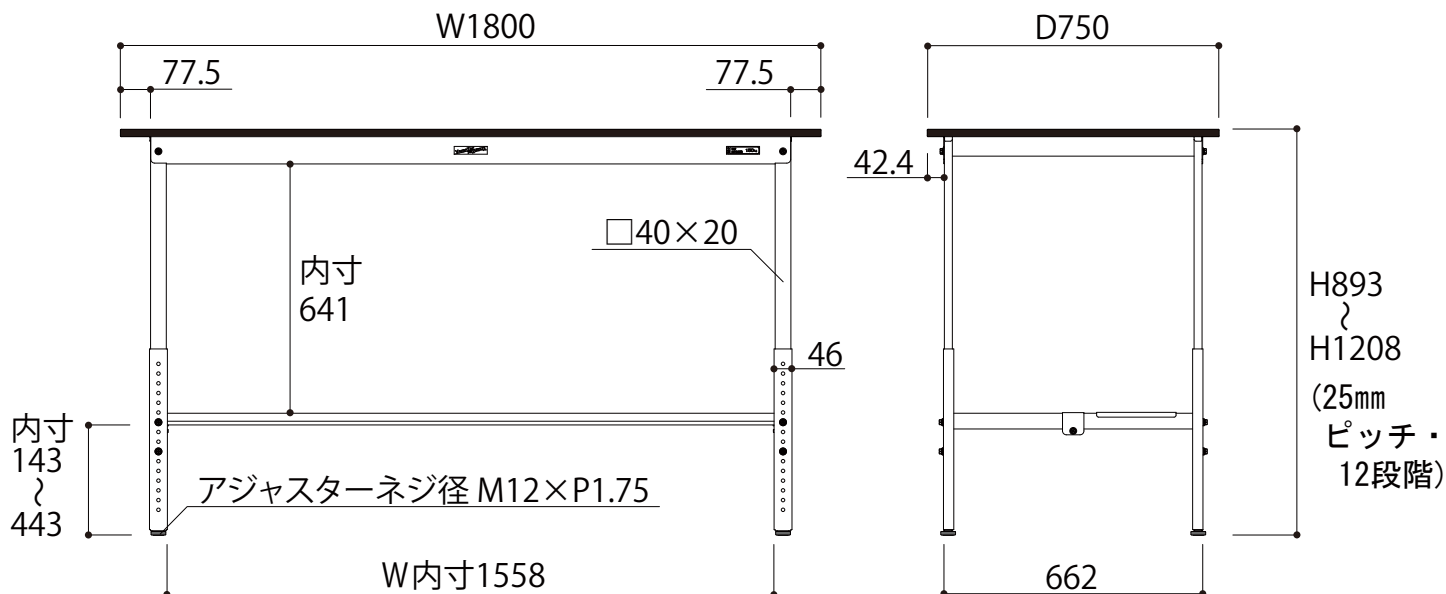
正面図
