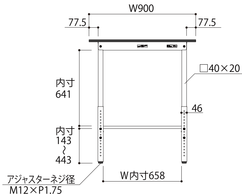
正面図
