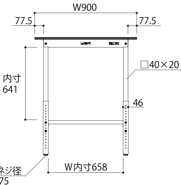
正面図
