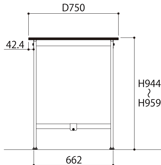
側面図
