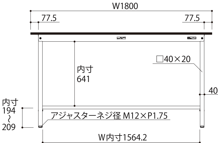
正面図
