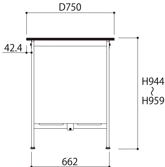
側面図
