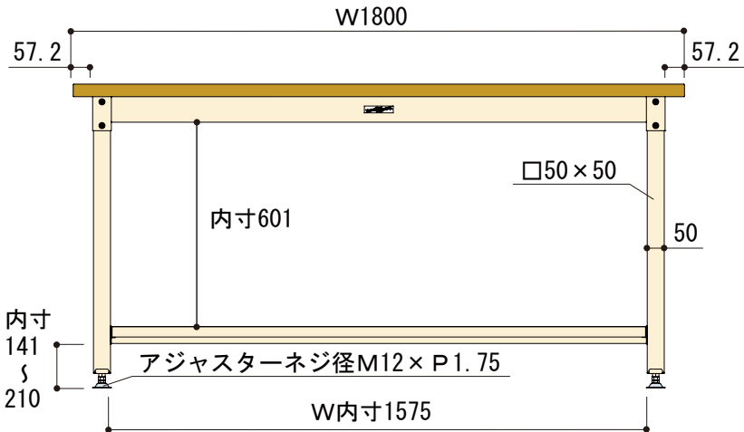
正面図
