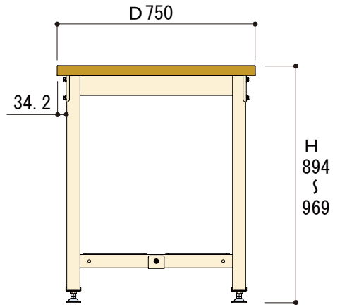
側面図
