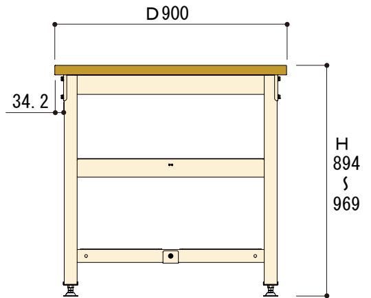
側面図
