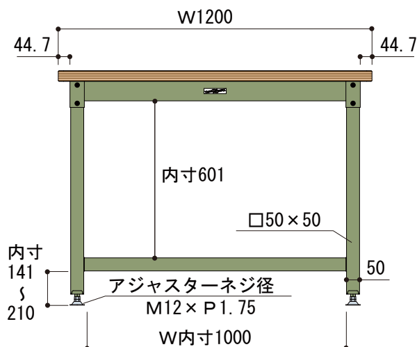
正面図
