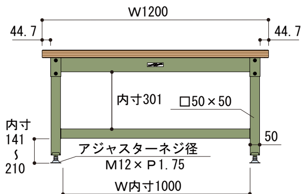
正面図
