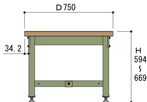
側面図
