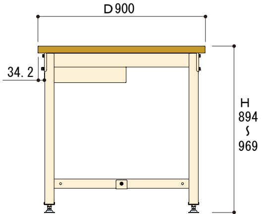
側面図
