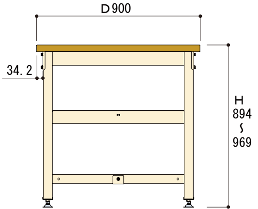
側面図
