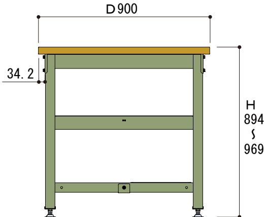
側面図
