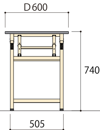
側面図
