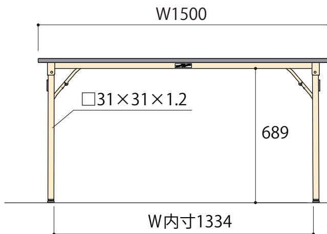
正面図
