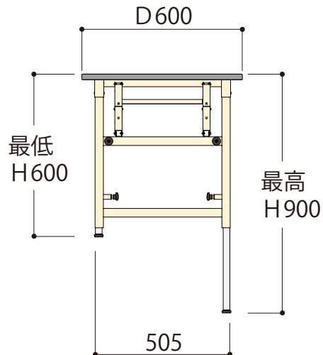
側面図
