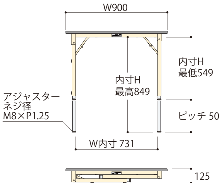
正面図
