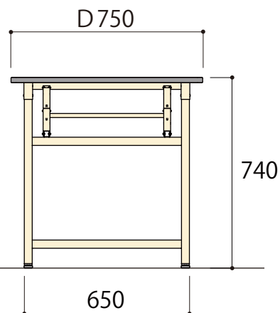
側面図
