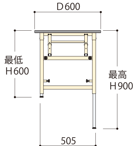
側面図
