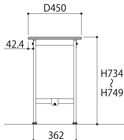
側面図
