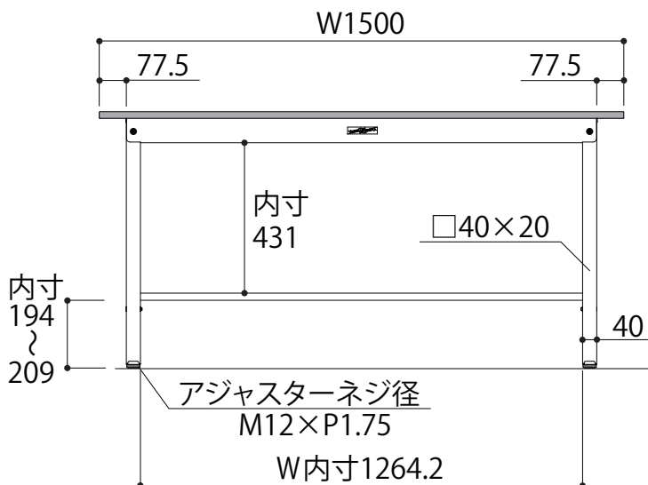
正面図
