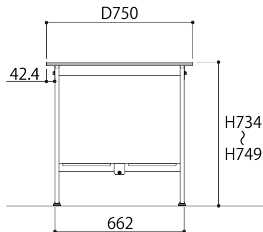
側面図
