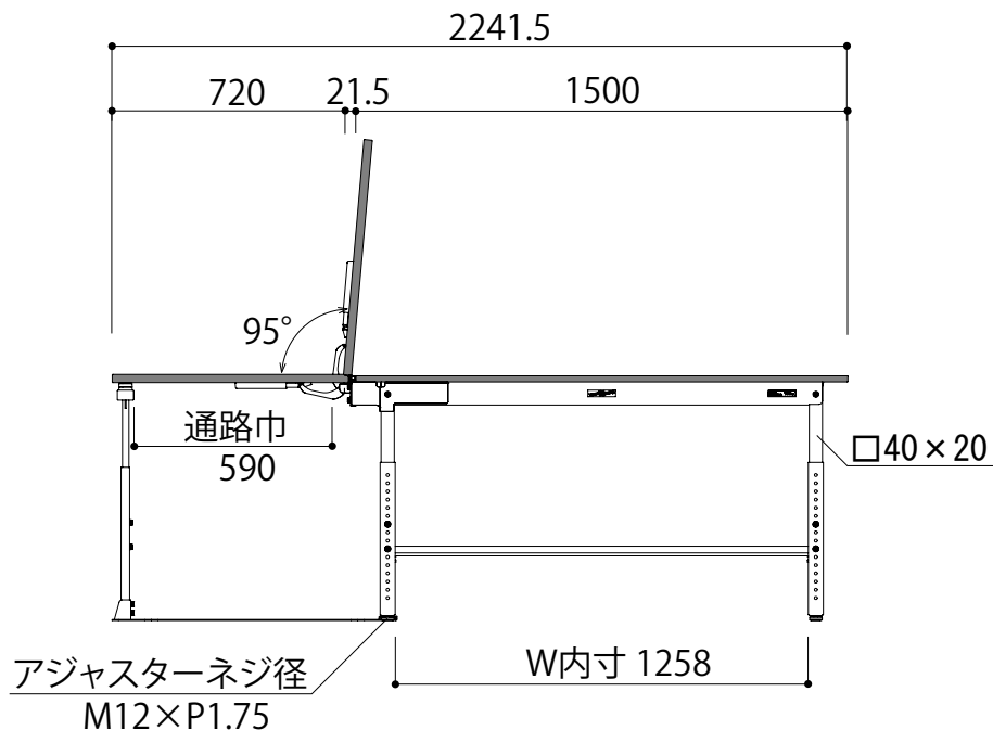
正面図
