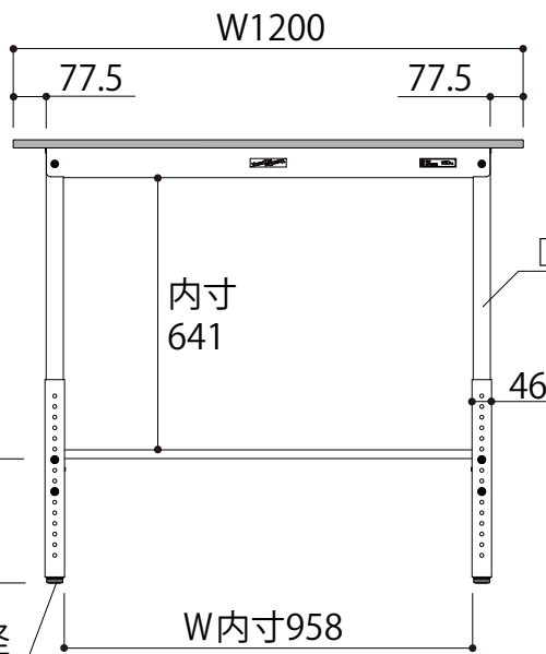
正面図
