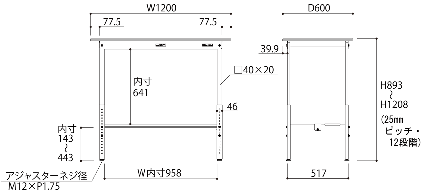
正面図
