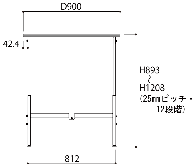
側面図
