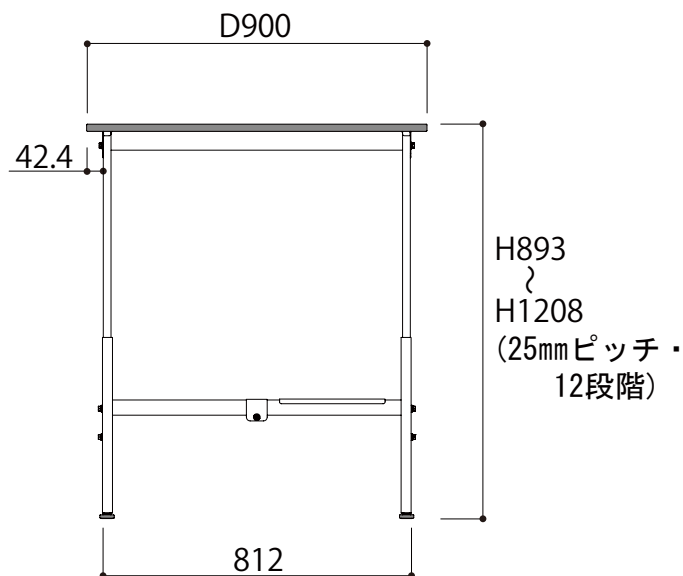
側面図
